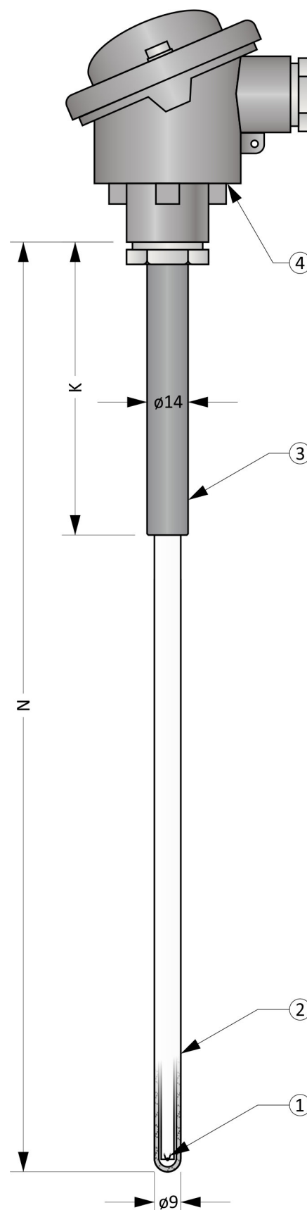
Obrázek 6MA.1: MTC6MA
